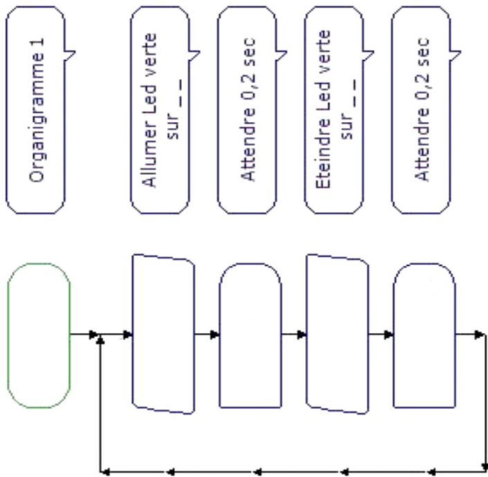
Organigramme1 Permet de faire clignoter la Led verte avec un temps de 0,2 seconde
