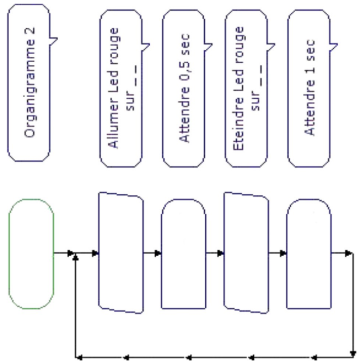
Organigramme2 Permet de faire clignoter la Led rouge Allumage pendant 0,5 sec, Extinction pendant 1 sec :
