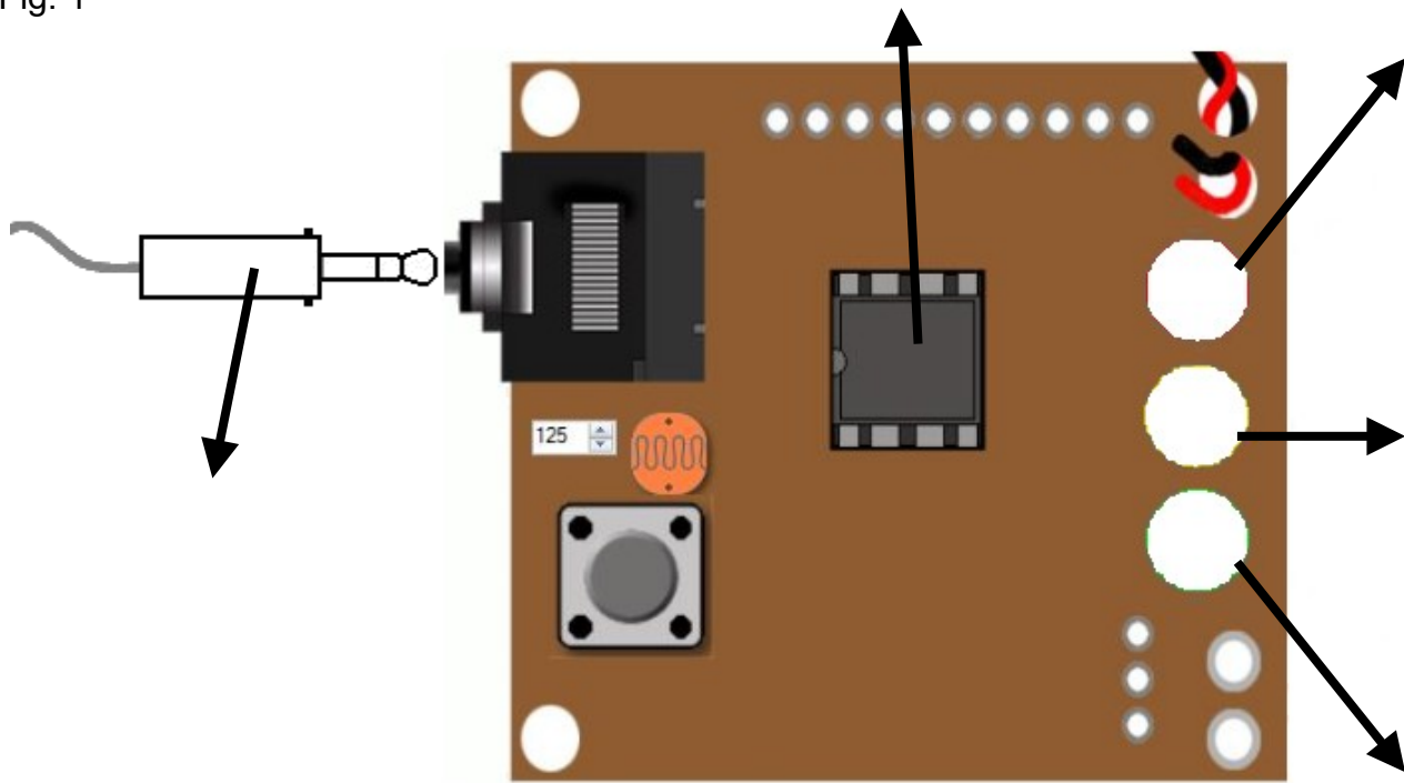
Simulateur : AXE130 Simple PIC Kit
