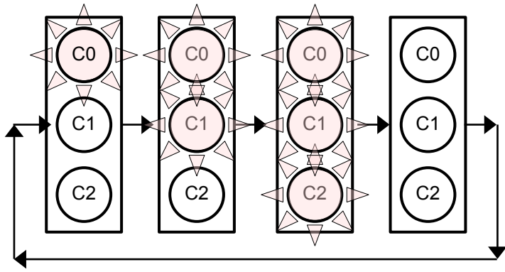
Organigramme3 Permet d'allumer la led rouge, puis la led jaune et enfin la led verte. Tout éteindre et recommencer
